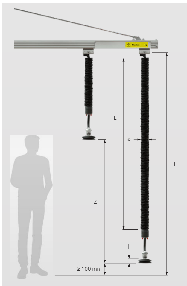
Z: slanglängd (mm) H: standard installationshöjd ca 2900 mm h: höjd sugfot / lyftok (mm) ca 50-120 mm ø: diameter lyftslang (mm) L: längd lyftslang (mm)
