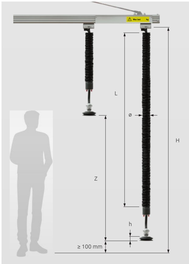
Z: Schlauchlänge (mm) H: Standard-Installationshöhe ca. 2.900 mm H: Höhe Sauggreifer/Hubtraverse (mm) ca. 50-120 mm Ø: Durchmesser des Hubschlauchs (mm) L: Länge des Hubschlauchs (mm)
