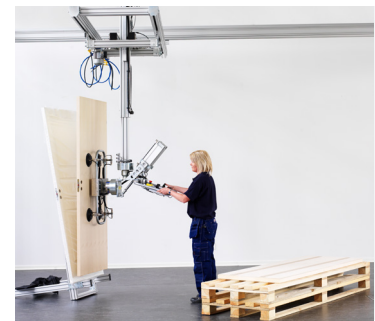
Préhenseur de porte
