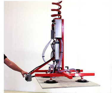
Ventouses pour panneaux
