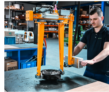
Préhenseur de moyeux
